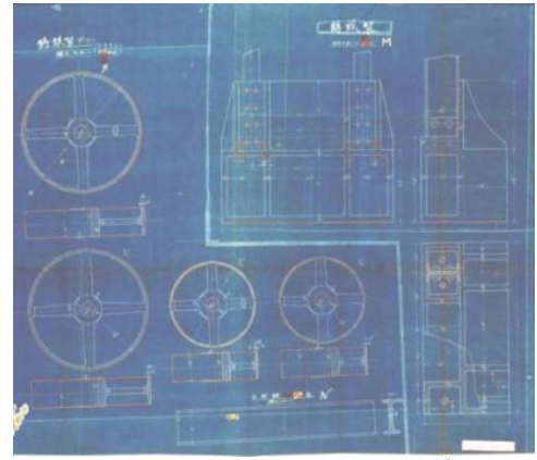
圖 2.4.61 葉煙草壓榨機用金具(鑄鉄製)
