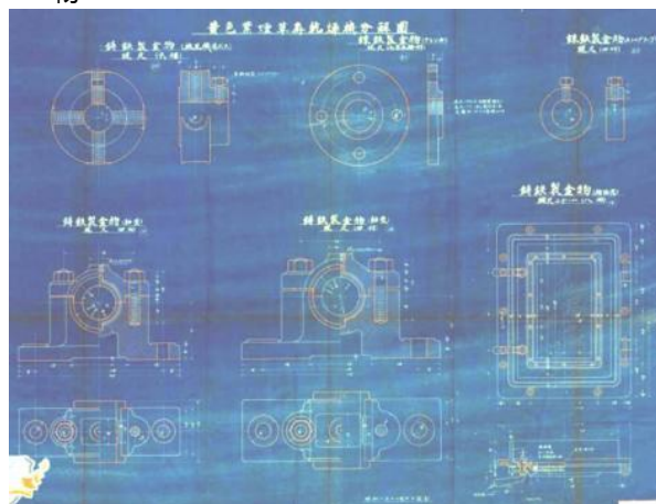
圖 2.4.51 黃色葉煙草再乾燥機分解圖-鑄鉄製金物、 鍛鉄製金物
