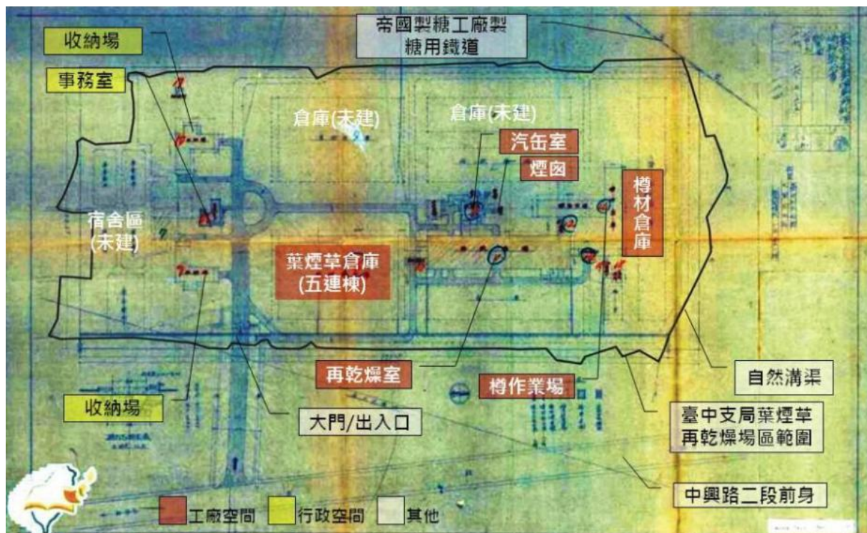
圖 2.4.190 昭和 16 年(1941)臺中支局葉煙草再乾燥場新築工事配置圖
