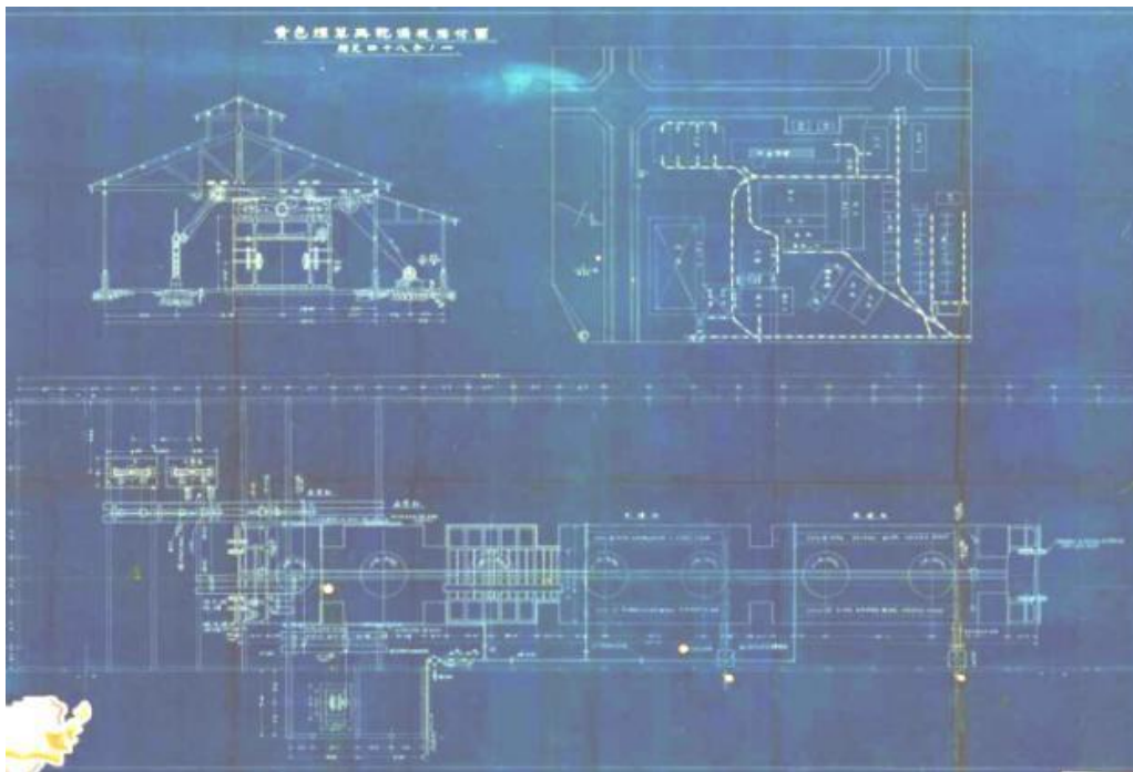
圖 2.4.44 黃色煙草再乾燥機据付圖
