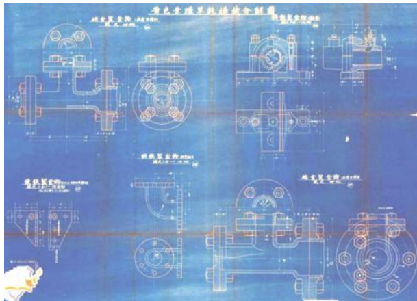
圖 2.4.56 黃色葉煙草乾燥機分解圖-鑄鉄製金物、鍊鉄 製金物、砲金製金物
