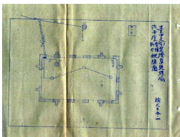
圖 2.4.183 臺中支局葉煙草再乾燥場汽缶室電燈動力配線圖
