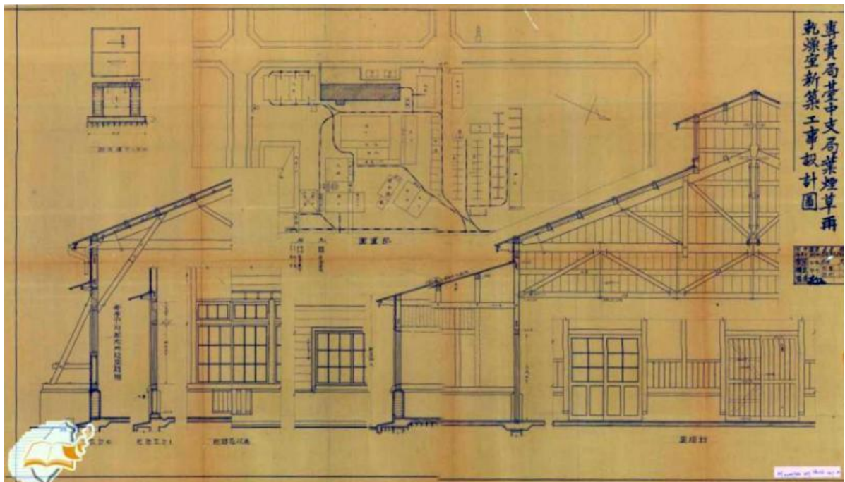
圖 2.4.30 昭和 8 年(1933)專賣局臺中支局葉煙草再乾燥室新築工事設計圖
