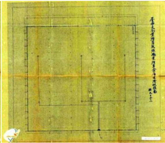
圖 2.4.186 臺中支局葉煙草乾燥場葉煙草倉庫(五連棟)電燈配置圖
