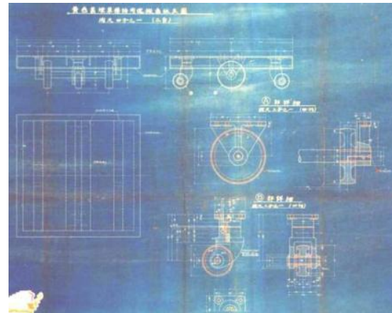
圖 2.4.57 黃色葉煙草樽詰用運搬車組立圖
