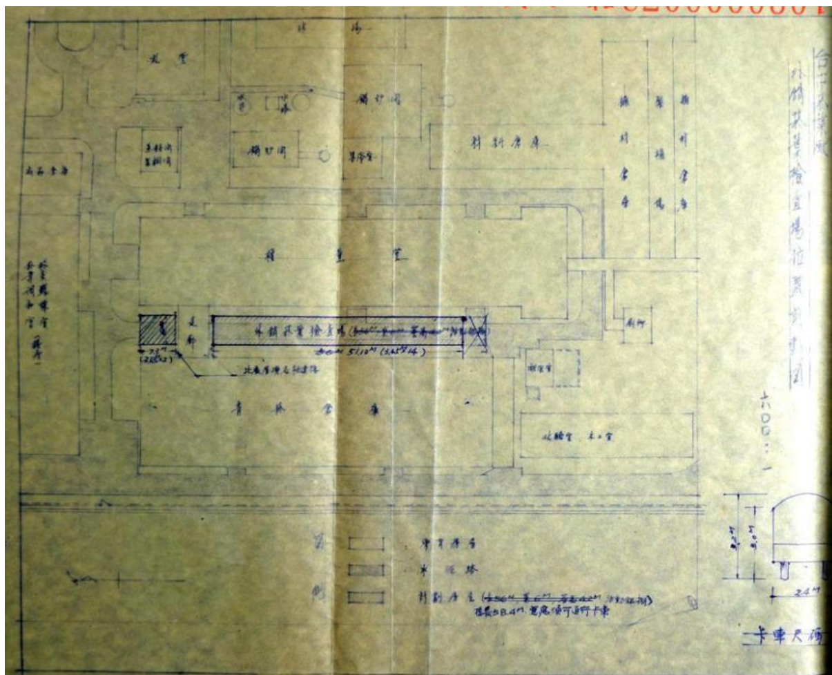
圖 2.4.318 民國 51 年(1962)4 月 4 日臺中菸葉廠上呈臺灣省菸酒公賣局請求同意增建外銷青菸檢查用鋁棚公文附圖-外銷青菸檢查場位置圖
