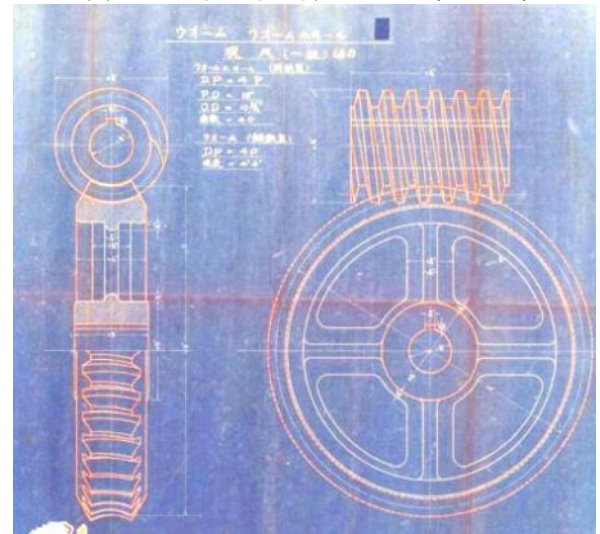
圖 2.4.63 黃色種葉煙草再乾燥機ウオーム、ウオームホイール(一組)(鉄製金物、鋼鉄製金物)
