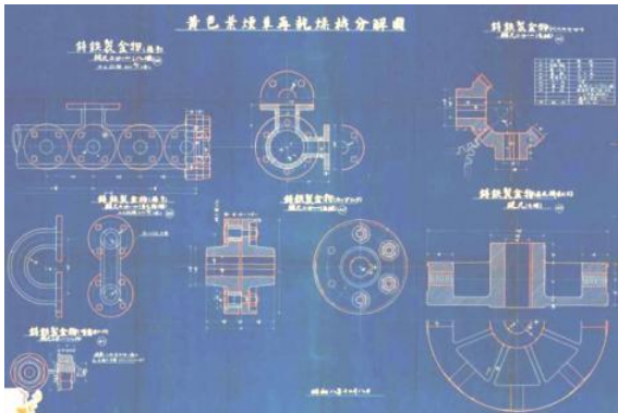
圖 2.4.54 黃色葉煙草再乾燥機分解圖-鑄鉄製金物
