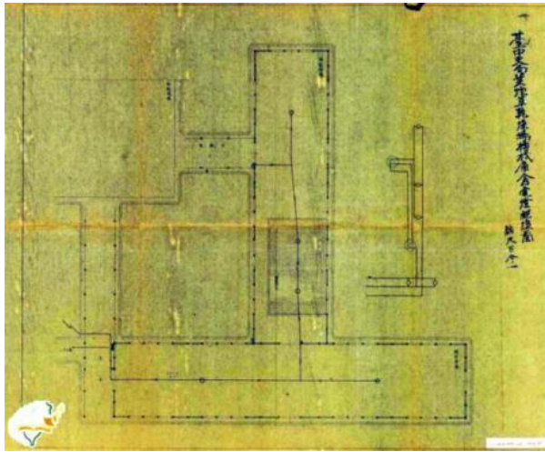
圖 2.4.185 臺中支局葉煙草乾燥場樁材庫舍電燈配線圖
