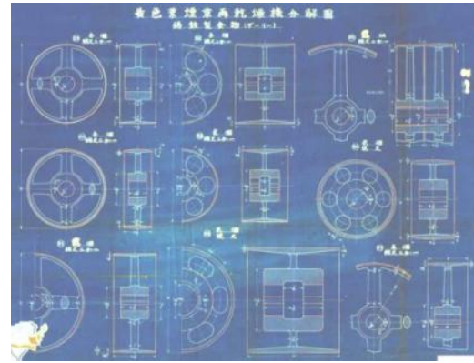
圖 2.4.53 黃色葉煙草再乾燥機分解圖-鑄鉄製金物 プーリ
