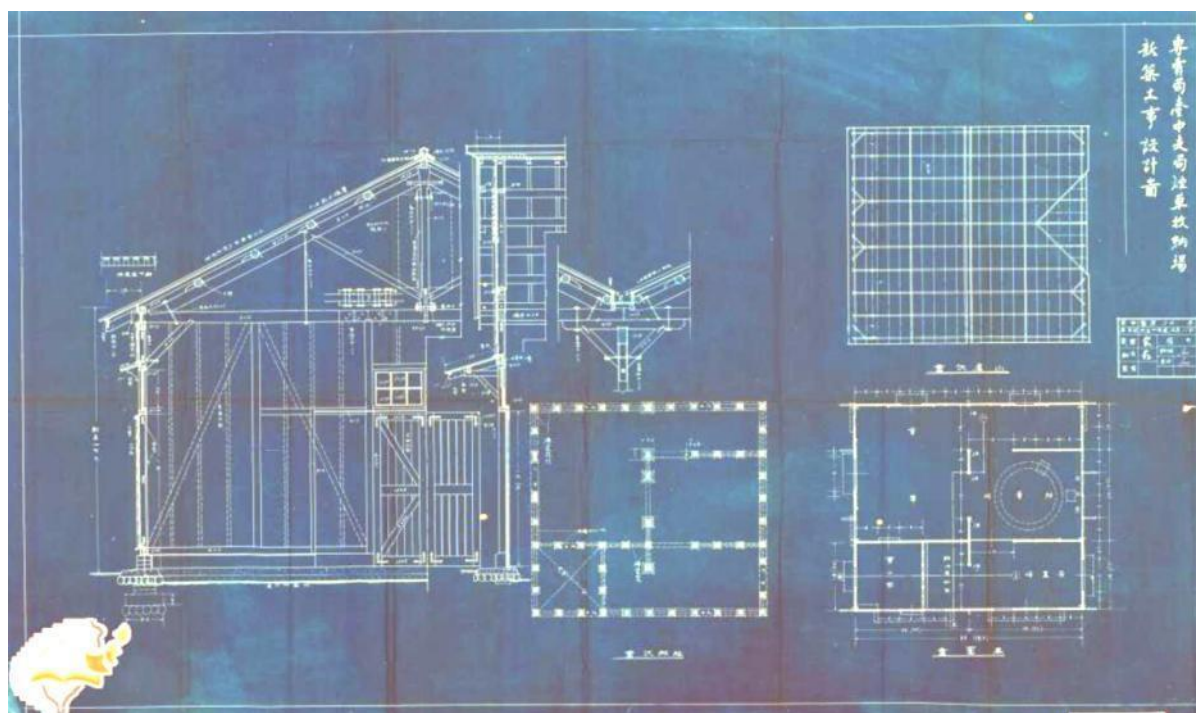
圖 2.4.16 大正 15 年(1926)臺中支局葉煙草收納場新築工事設計圖
