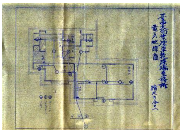
圖 2.4.182 臺中支局葉煙草再乾燥場事務所電氣配線圖
