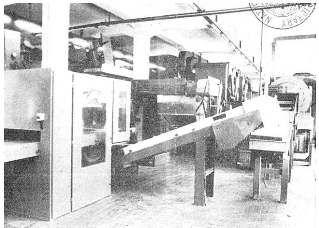
圖 2.4.405 新型除骨機照片 資料來源：《臺菸月刊 14：9》，封面
