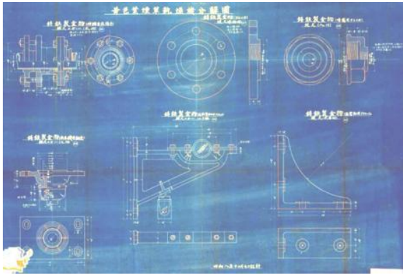
圖 2.4.52 黃色葉煙草乾燥機分解圖-鑄鉄製金物
