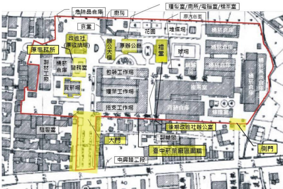
圖 2.4.205 行政管理空間建築物分布示意圖
