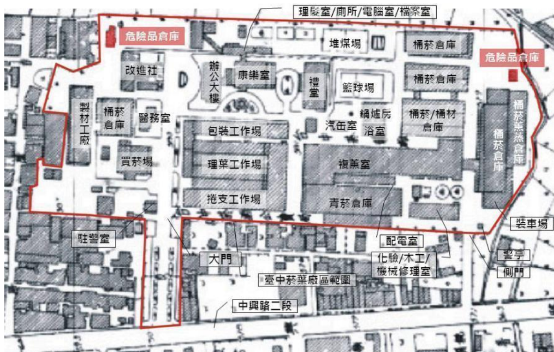
圖 2.4.199 民國 59 年(1970)《臺中市地形圖》局部-臺灣省菸酒公賣局臺中菸葉廠區危險品倉庫分布示意圖
