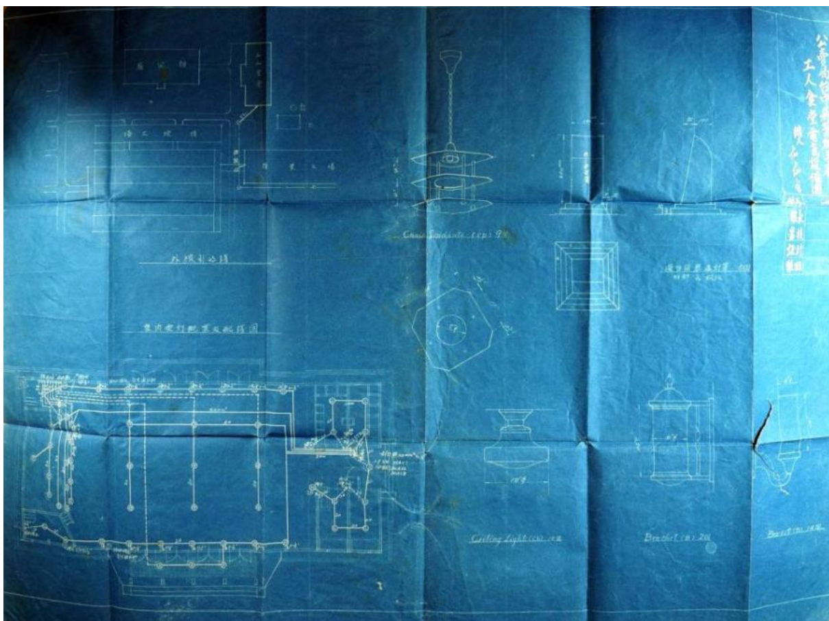
圖 2.4.238 民國 41 年(1952)7 月臺中菸草工場上呈設計圖面、預算書、工程說明書公文附圖之一-《工人食堂電氣設備圖》
