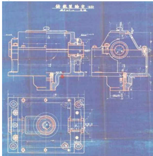
圖 2.4.64 黃色種葉煙草再乾燥機-鑄鉄製軸受
