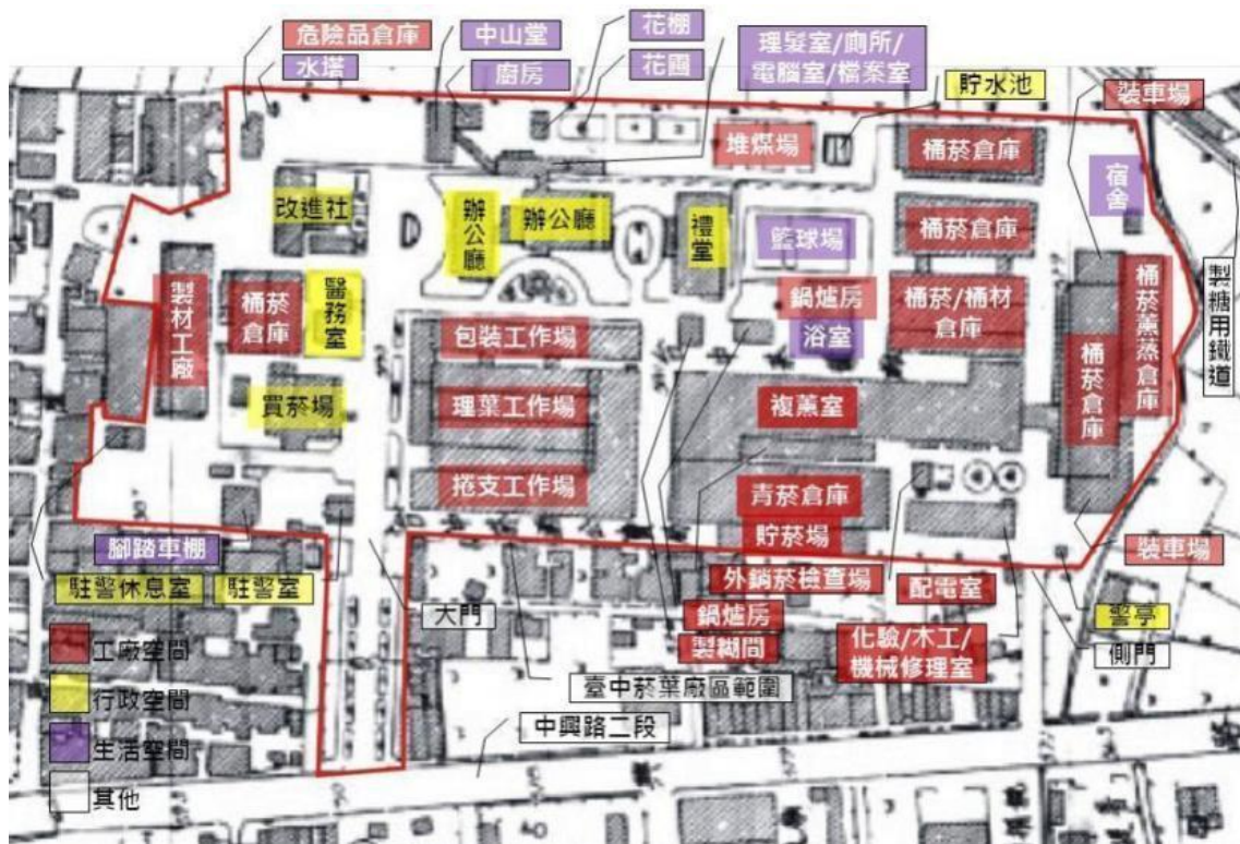
圖 2.4.203 民國 59 年(1970)《臺中市地形圖》局部-臺灣省菸酒公賣局臺中菸葉廠區建築物分布示意圖 資料來源：本計畫以臺灣百年歷史地圖為底圖；本計畫標註
