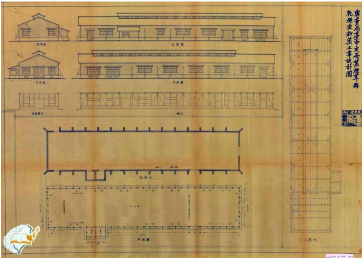
續圖 2.4.30 昭和 8 年(1933)專賣局臺中支局葉煙草再乾燥室新築工事設計圖
