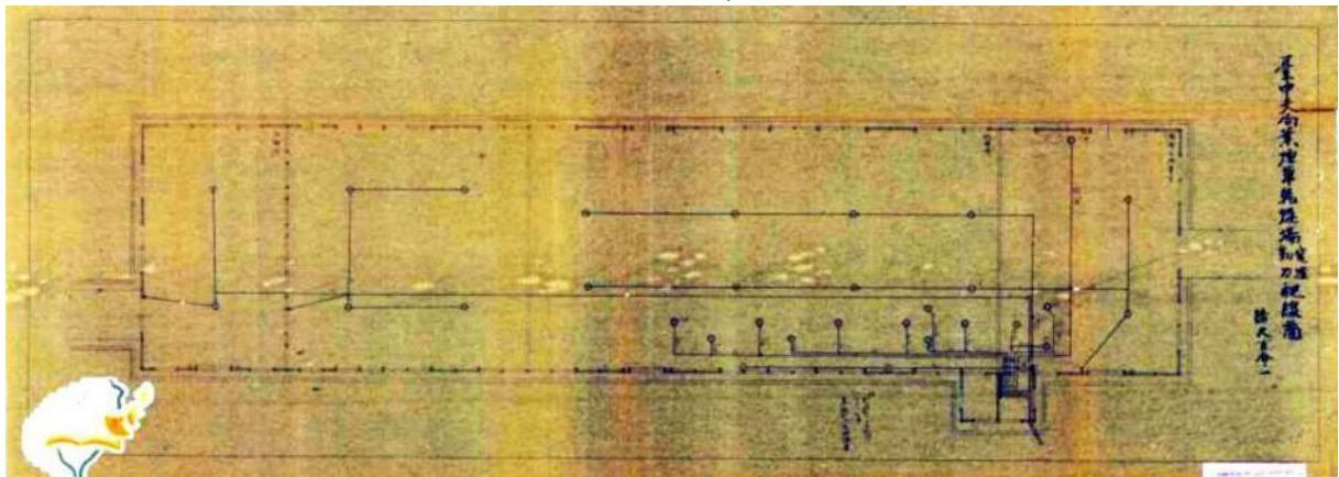
圖 2.4.187 臺中支局葉煙草乾燥場電燈動力配線圖
