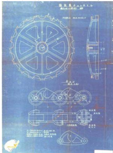
圖 2.4.62 黃色種葉煙草再乾燥機(鑄鉄製チェンホイール)
