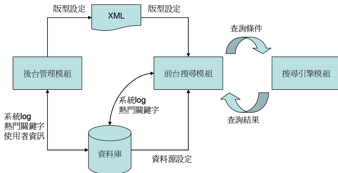
圖 6 系統整體程式結構圖
