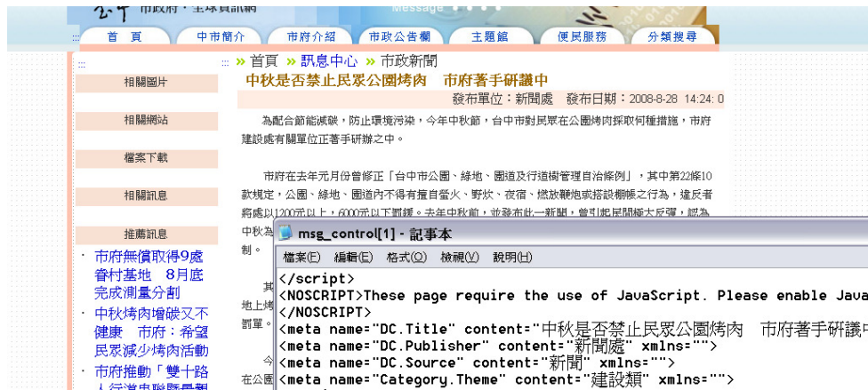
圖 1 0 市政新聞運用網頁 HTML Meta Tag 解決新聞分類問題
