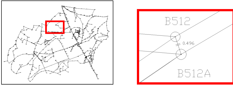
圖 5 近似坐標給定不佳網形例
