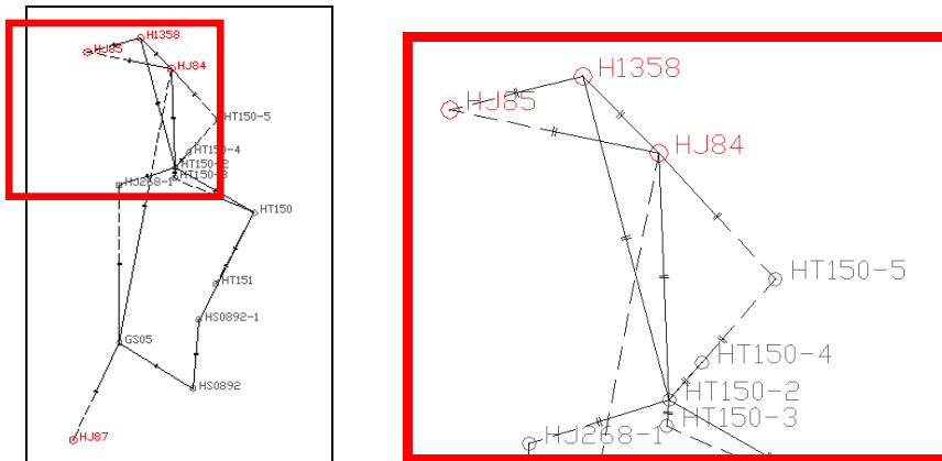
圖 3 點號輸入錯誤網形例
